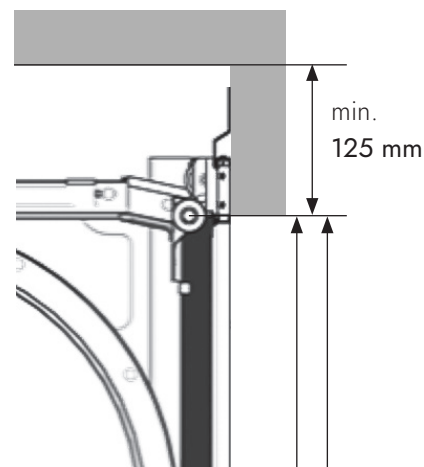
■ VÝŠKA VRAT = OTVOR
