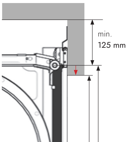
■ VRATA VYŠŠÍ NEŽ OTVOR
