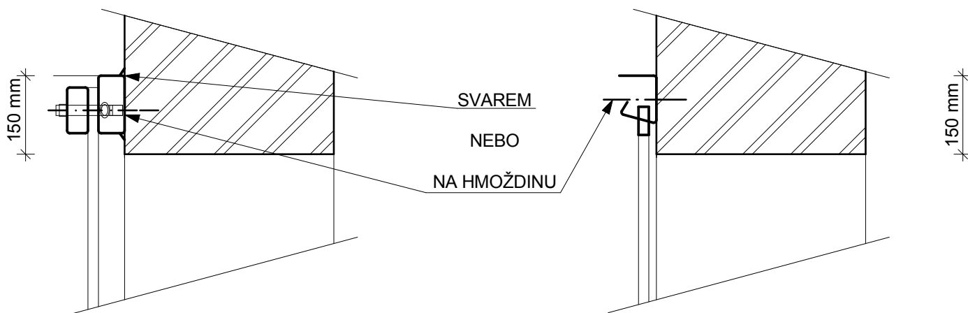
SVĚRNÁ LIŠTA -TYP B (nad světlost otvoru)
