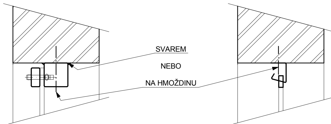
SVĚRNÁ LIŠTA -TYP A (do světlosti otvoru)
